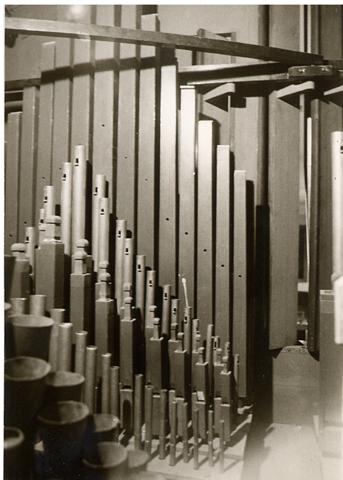
La console et trois vues de la tuyauterie du GO. Les jalousies de la boîte expressive étaient encore en arrière de la façade. En allant vers l'avant : Montre (en façade) Flûte traversière, Gambe, Bourdon, Prestant, chape vide, Flûte 4, Doublette 2, hautbois 8, Clairon 4.
