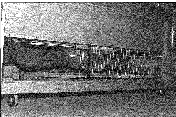
Sommier et mécanique de Pédale.
