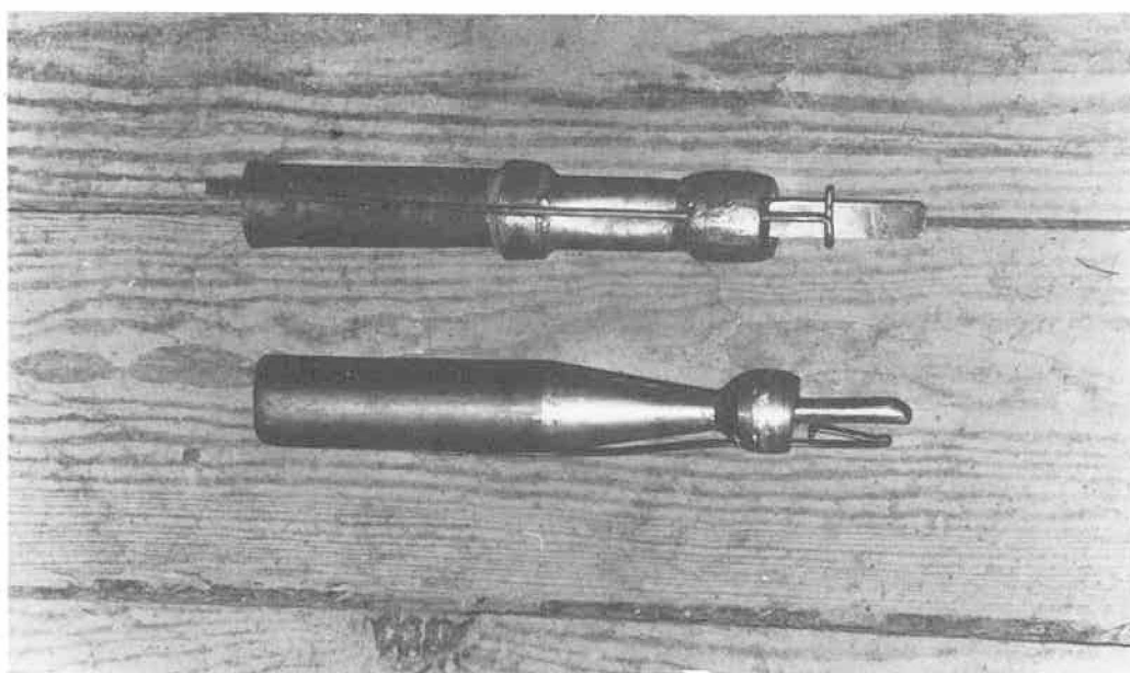
Tuyaux d'anches (détail du noyau et du canal d'anche)
