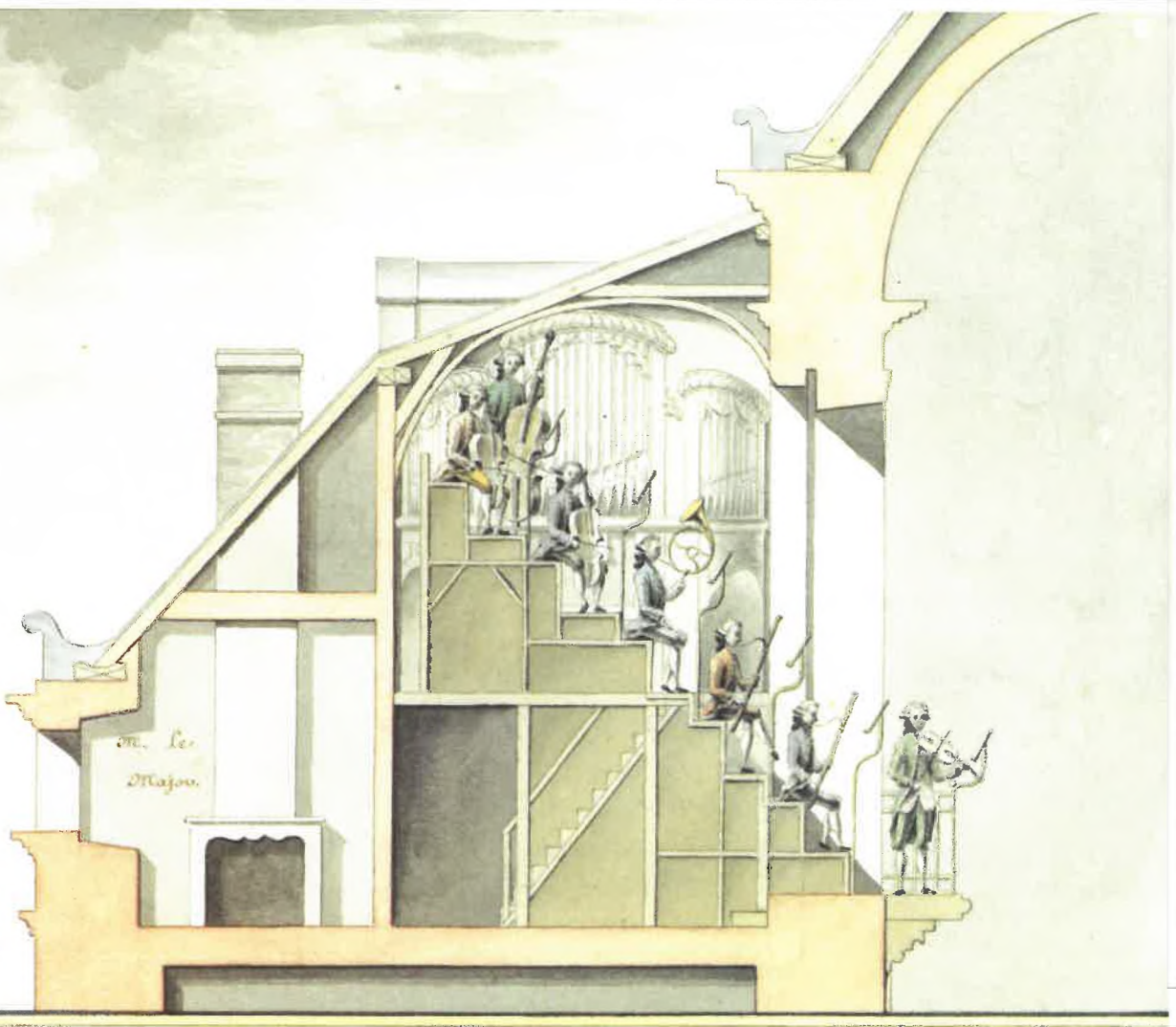
COUPE de la nouvelle Tribune.
