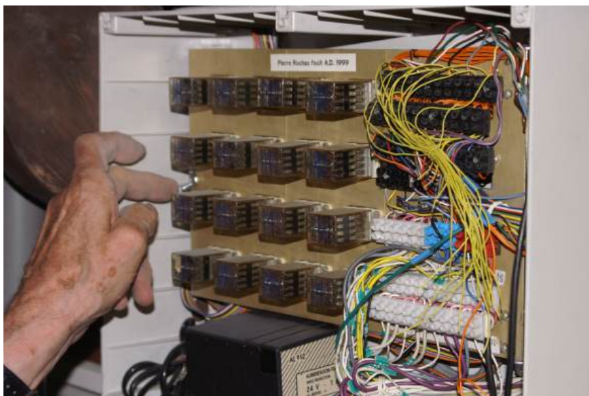
Commandes électriques des extensions de pédale coté C à l'intérieur du buffet
