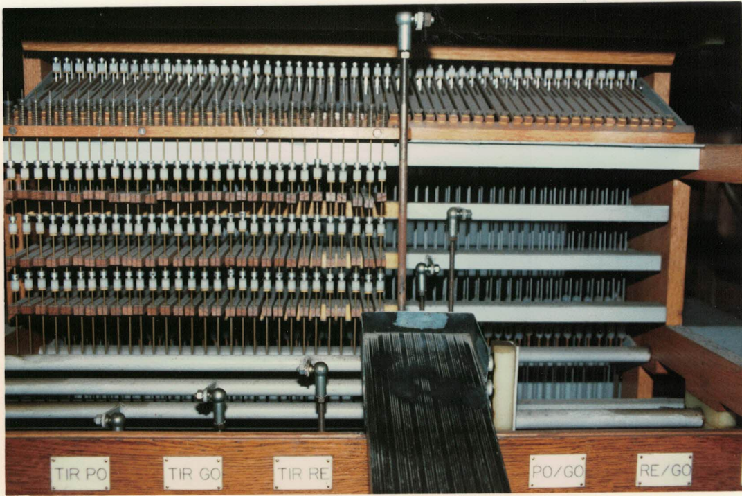
CONSOLE - PARTIE INFÉRIEURE OUVERTE : ACCOUPLEMENTS ET TIRASSES (VUE DEPUIS LE PÉDALIER)
