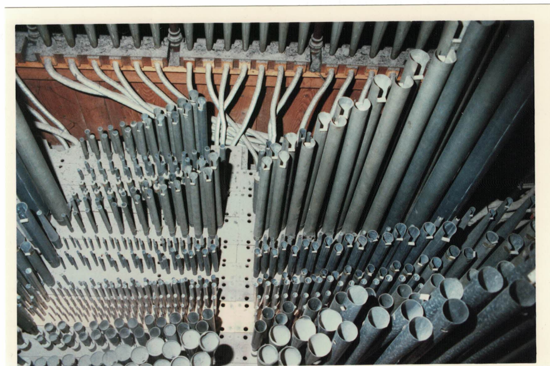
INTERIEUR DU POSITIF ↴
